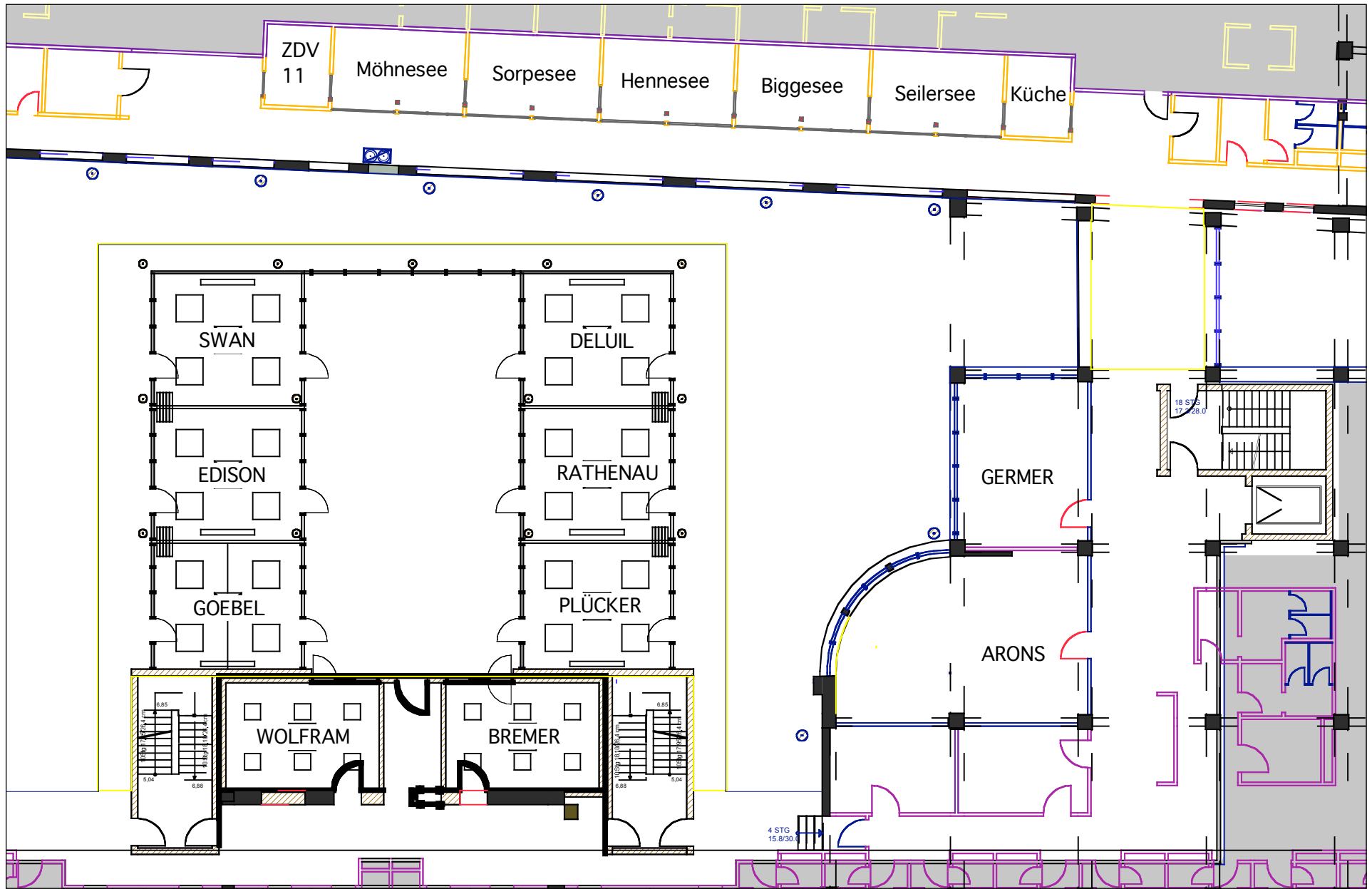
1. Obergeschoss
